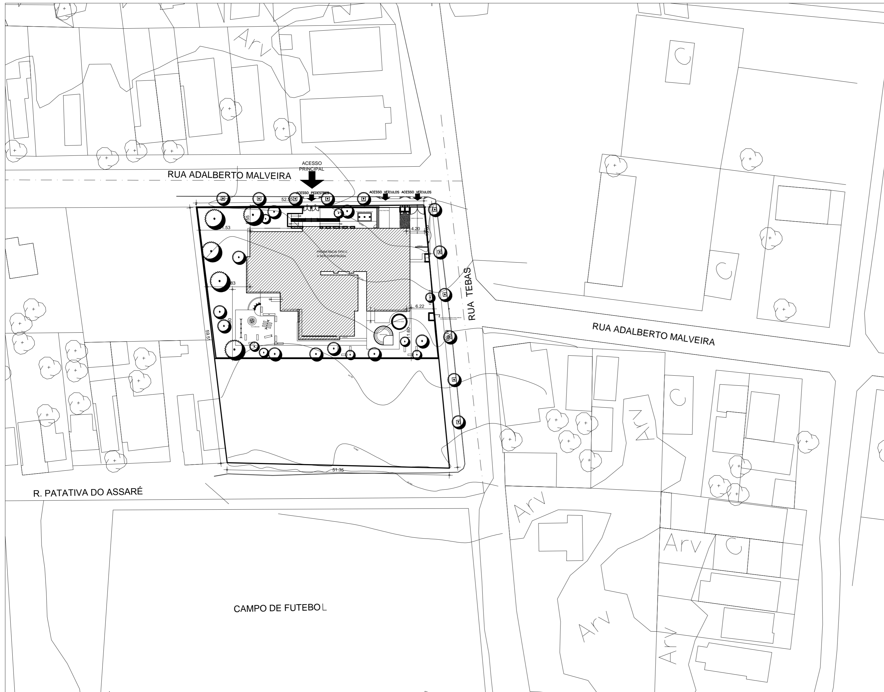
1 PLANTA DE SITUAÇÃO ESC.: 1:500
